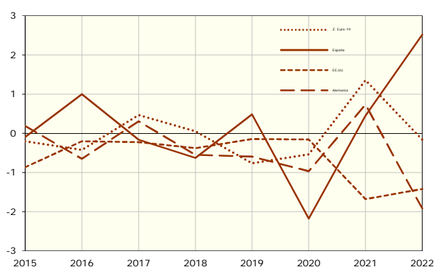
DEMANDA EXTERNA
