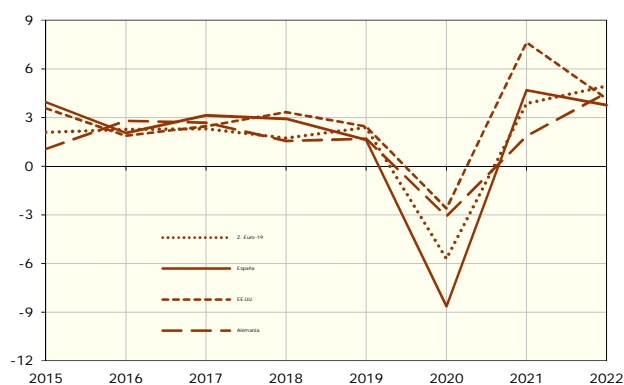
DEMANDA NACIONAL
